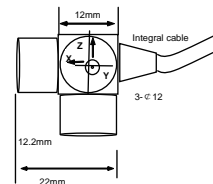
ULT2122、ULT2123 ULT2124 外形尺寸图
