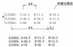
ULT2502 、ULT2503 ULT2504 外形尺寸图
